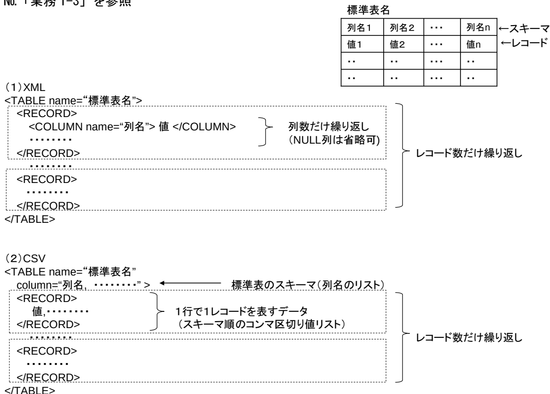
図 3. 2. 3 1 汎用検索インタフェースの結果例
