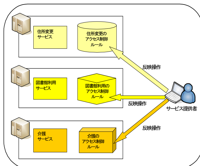
図 3. 5. 2 1 サービス提供者の問題点
