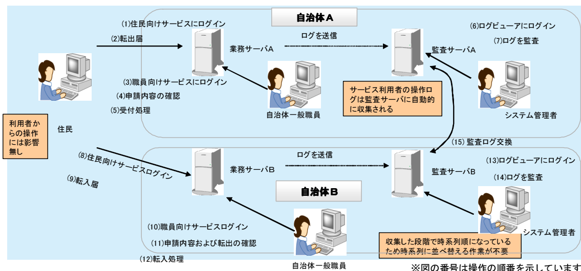
図 3. 5. 27 監査証跡取得機能の全体概要図
