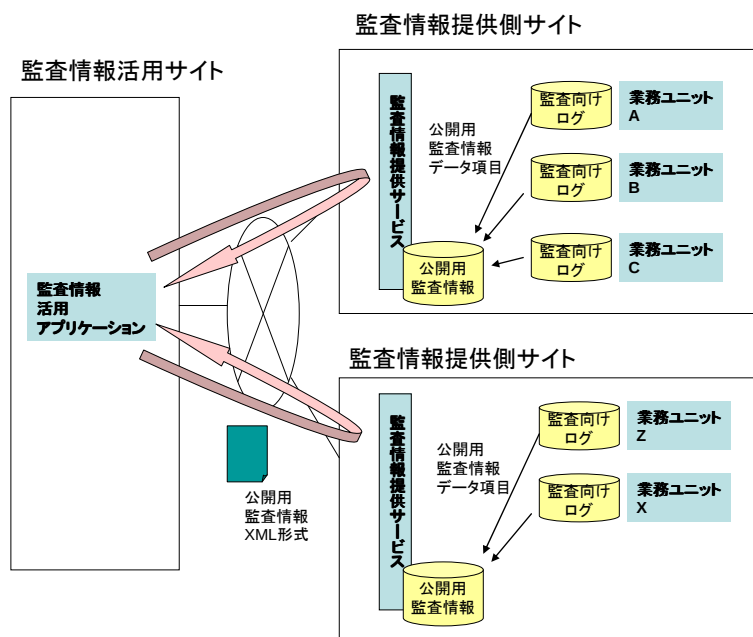
図3. 5. 29 監査証跡取得機能のシステム構成例
