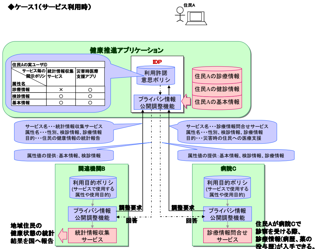
図3. 5. 25 プライバシ情報公開調整技術のユースケース図（サービス利用時）
