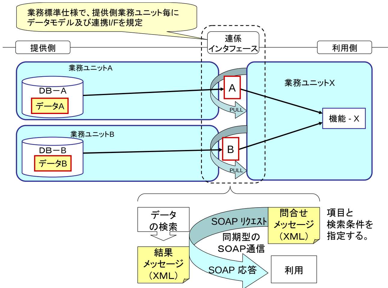
図 3. 2. 8 業務ユニット間の直接連携
