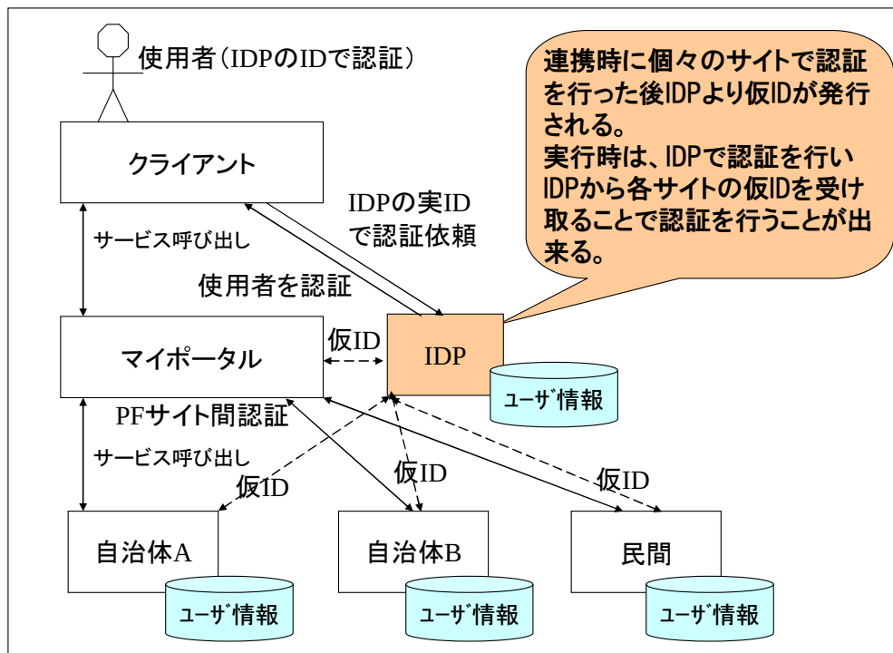
図3. 5. 20 プライバシ保護型認証連携技術
