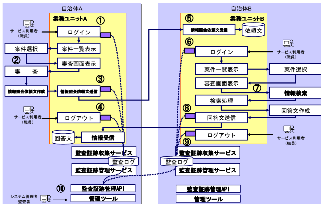
図 3. 5. 28 監査証跡取得機能でのユースケース図
