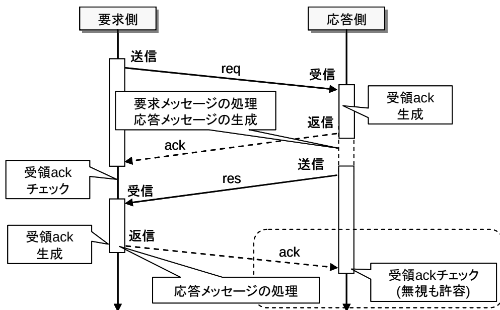
図3. 8. 6 リクエスト・レスポンス型同期型受領 Ack+非同期型レスポンス
