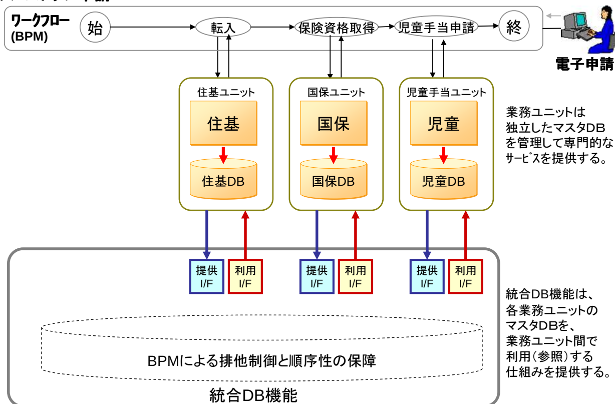
図3. 2. 5 統合DB機能の使い方(C方式)
