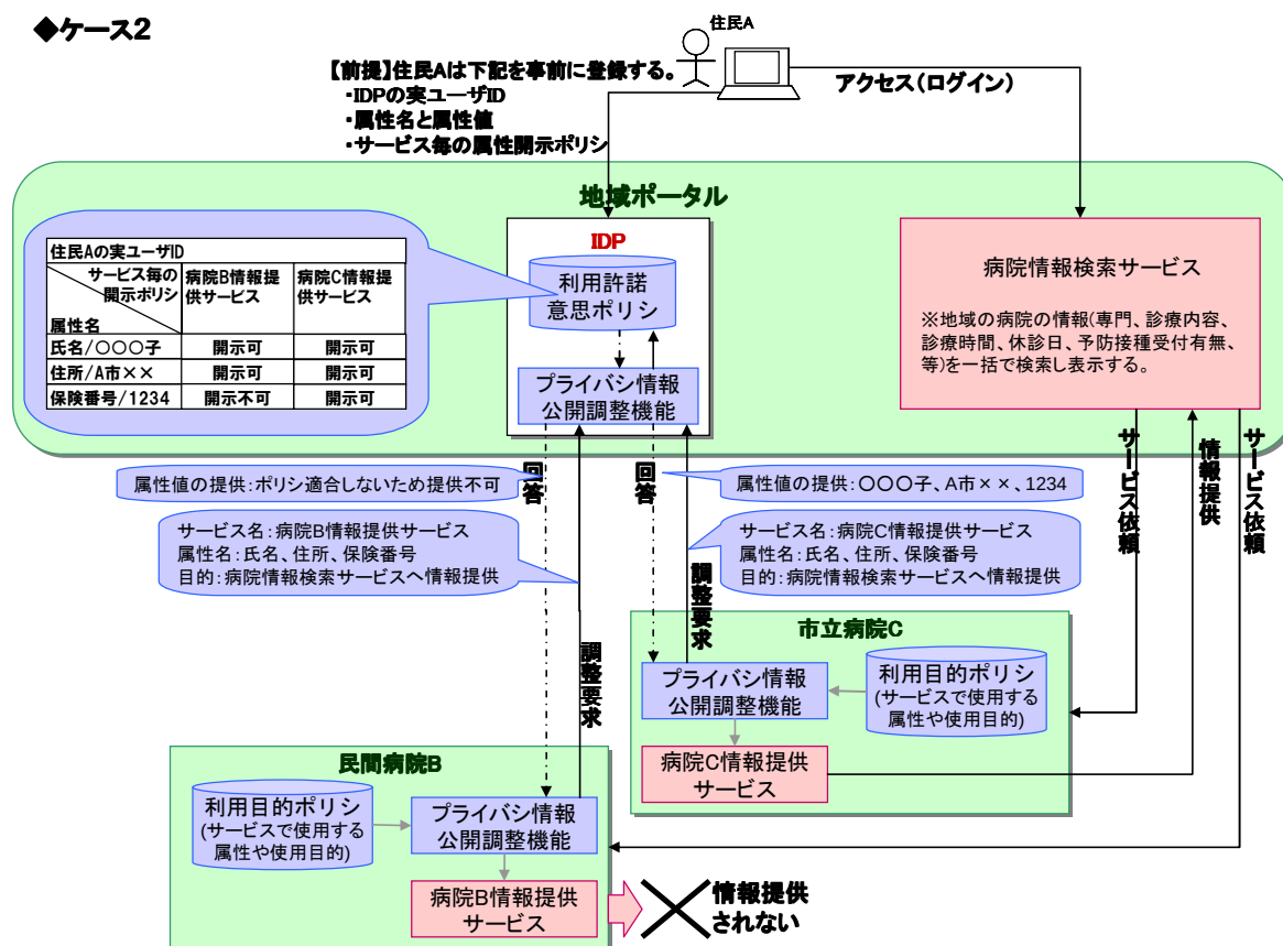
図3. 5. 26 プライバシ情報公開調整技術のユースケース図
