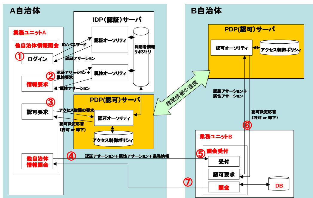
図3. 5. 2 2 権限管理基盤技術のユースケース
