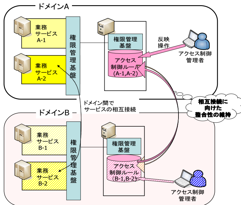
図3. 5. 24 権限情報同期技術のイメージ図
